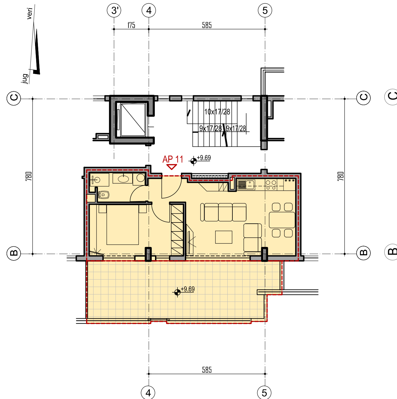
mobilm i apartamentit NR 11 (1+1) (kuota +9.69) sh 1:100
