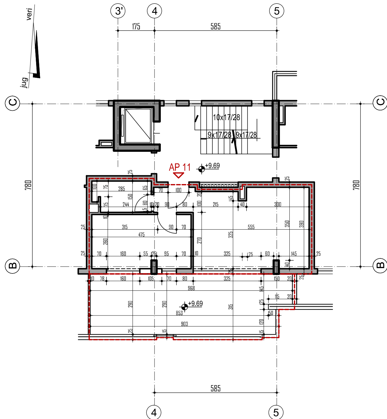
plan i apartamentit NR 11 (1+1) (kuota +9.69) sh 1:100
