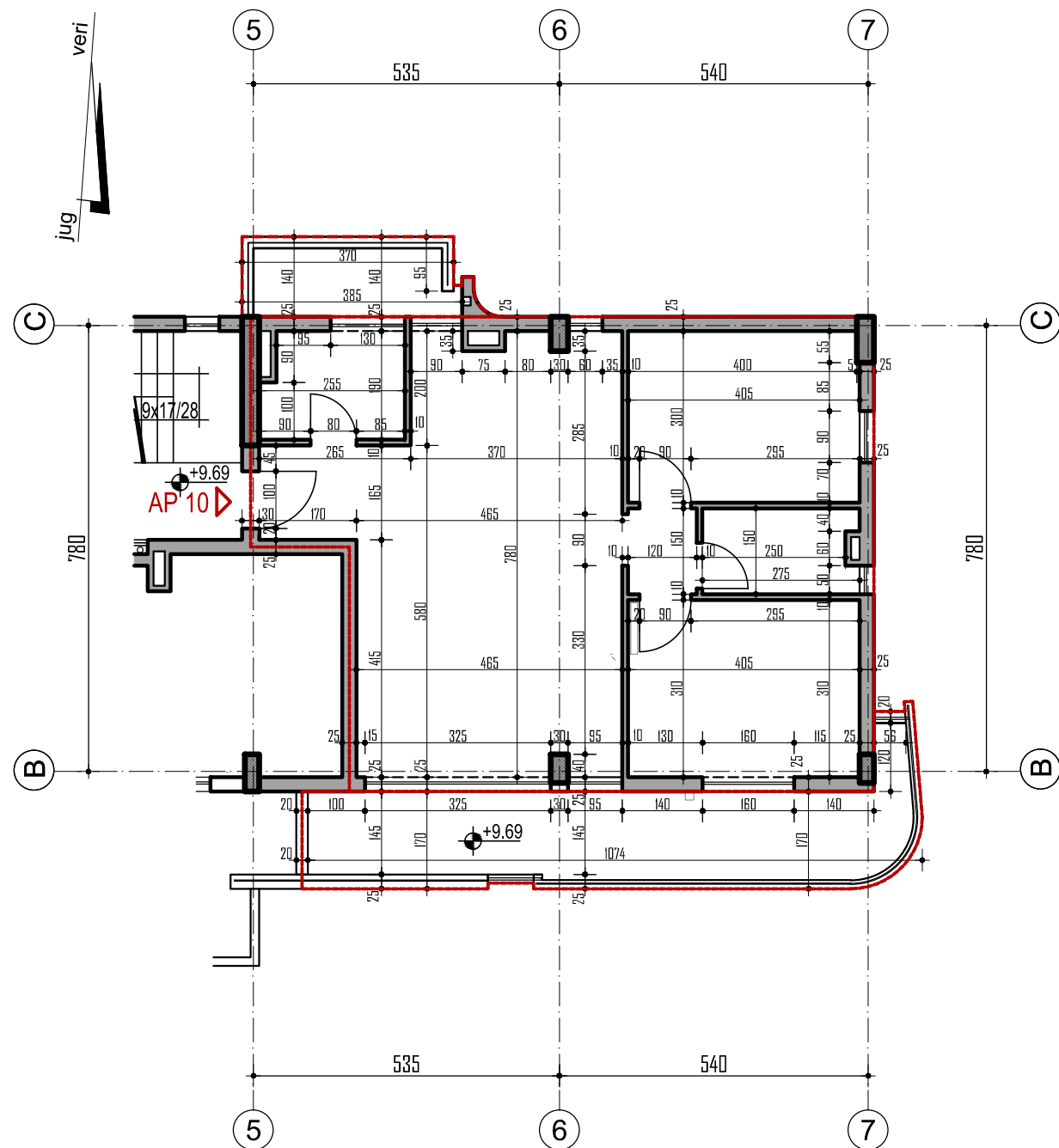
plan i apartamentit NR 10 (2+1) (kuota +9.69) sh 1:100
