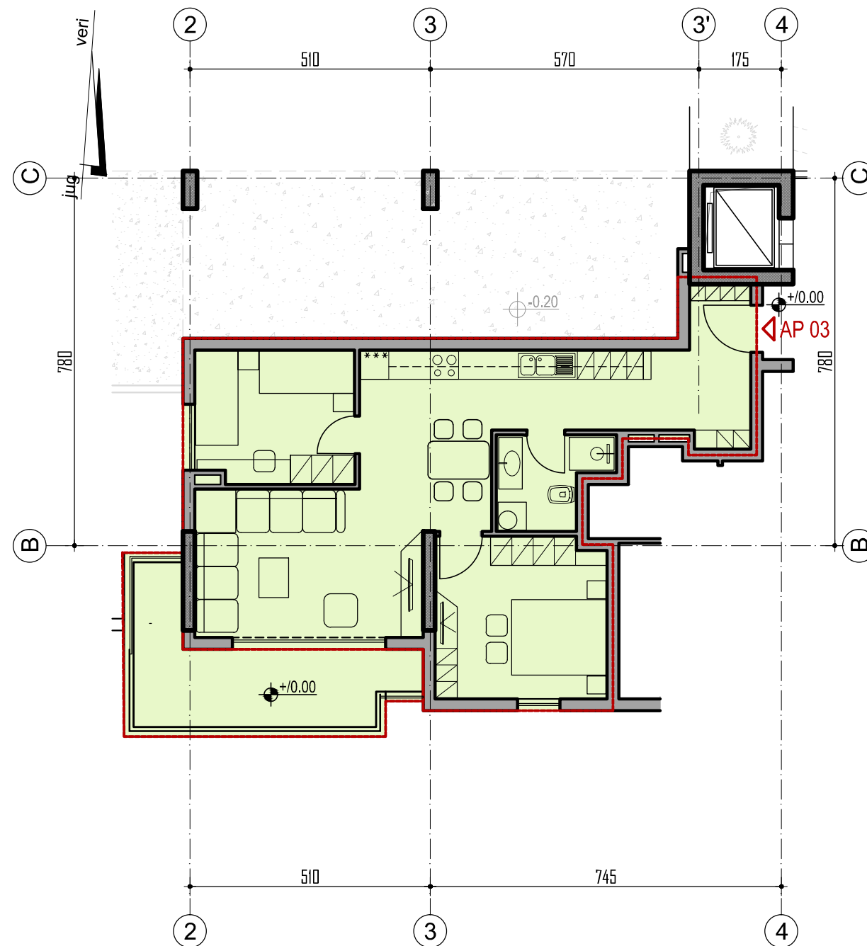
mobilm i apartamentit NR 03 (2+1) (kuota +/-0.00) sh 1:100
