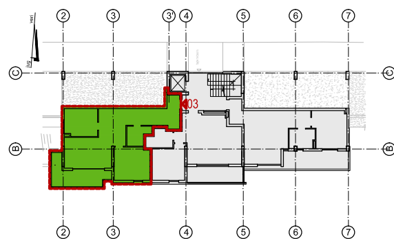
plan i katit në kuotën +/-0.00 apartamenti NR 03
