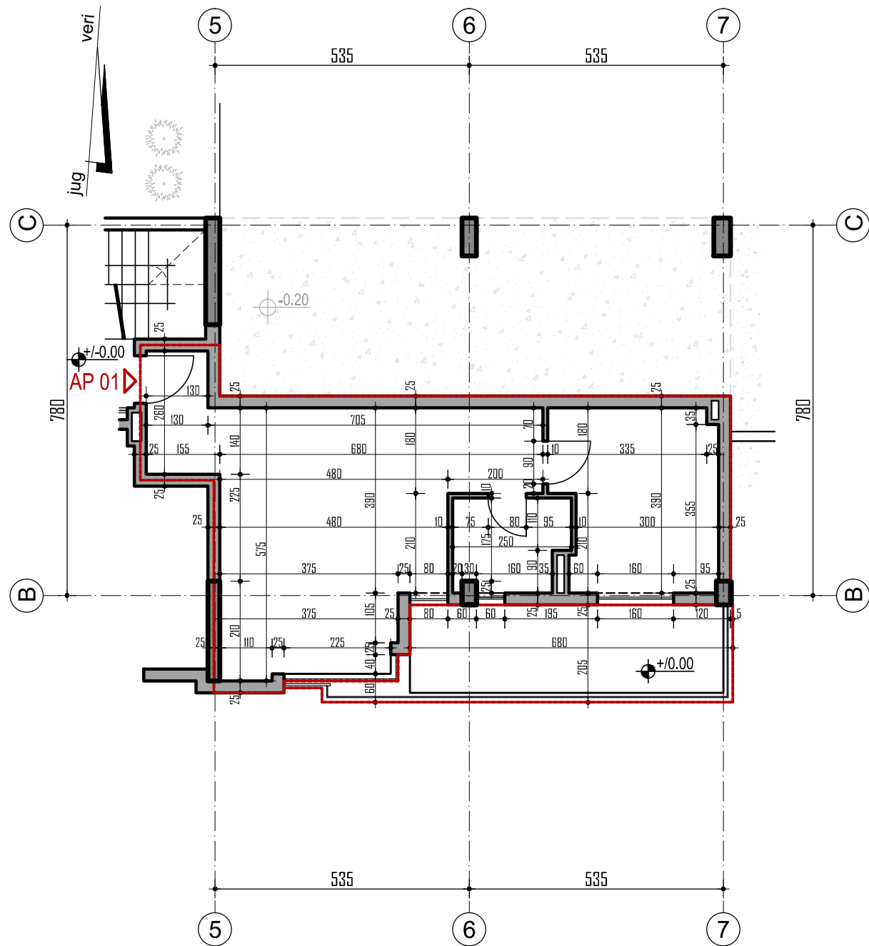
plan i apartamentit NR 01 (1+1) (kuota +/-0.00) sh 1:100
